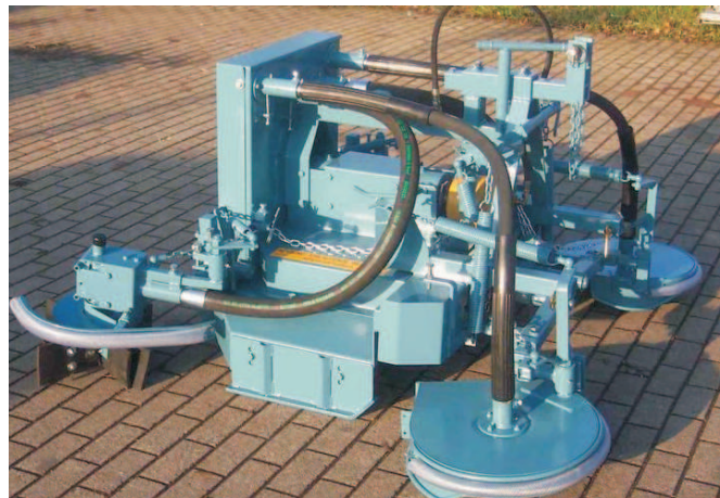
Komplettgerät HS 1200 Z mit angebauten Schwenscheiben und Stockputzern
